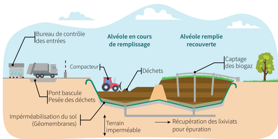
Schéma simplifié d'un centre d'enfouissement
